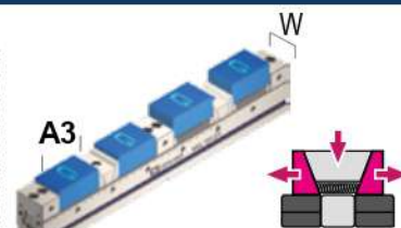
Art.613 - Ganascia mobile doppia di spinta (*Modelli predisposti per serrare 3 particolari)
